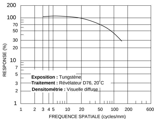
Courbe de modulation de transfert
